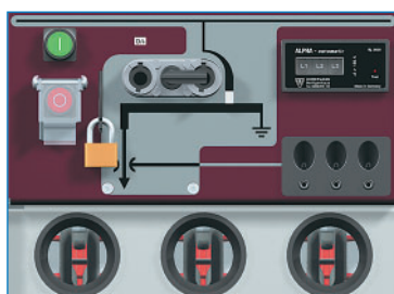
Заземленное положение.
